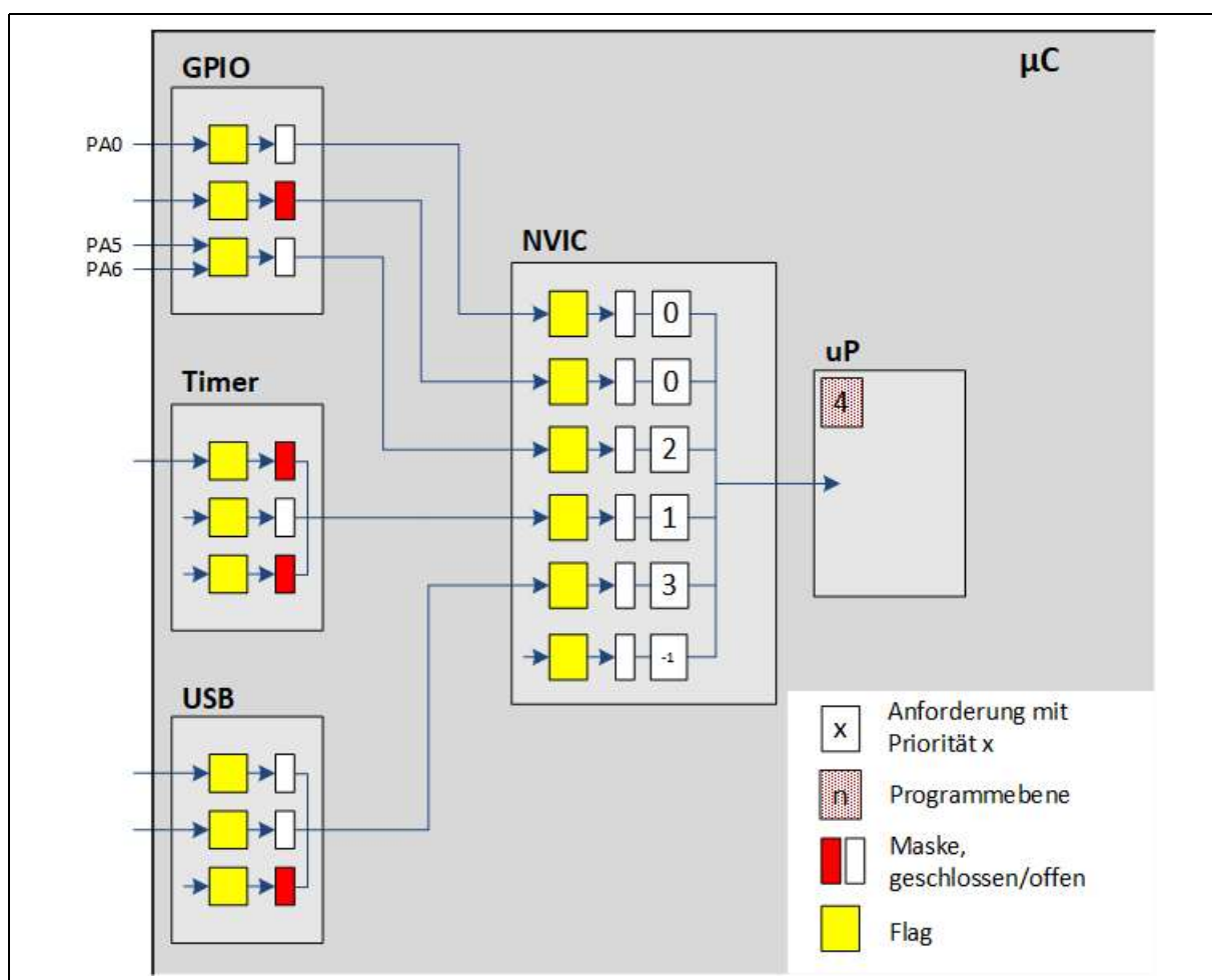
Abbildung 7: Typisches Interruptsystem eines \mu\text{C} mit ARM-Rechenkern
